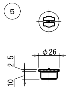
継手キャップ
